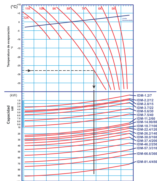
Evaporador Serie IDM
